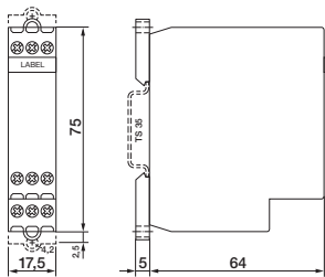
fig. 4. Dimensions (mm)
