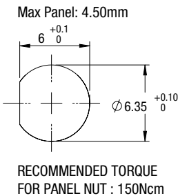
fig. 2. Abmessungen (mm)
