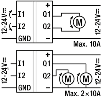
fig. 2. Function diagram
