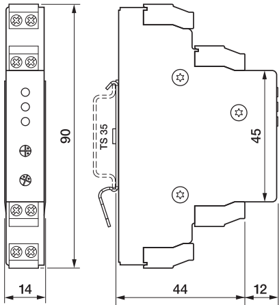
fig. 3. Dimensions (mm)
