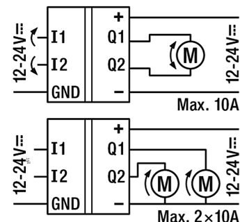
fig. 2. Funktionsdiagramm
