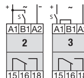
fig. 2. Wechselstrom-Schaltzyklen
