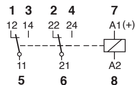
fig. 2. Wechselstrom-Schaltzyklen
