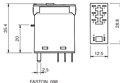
fig. 4. Dimensions (mm)
