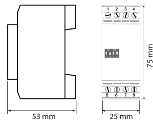
fig. 1. Abmessungen (mm)
