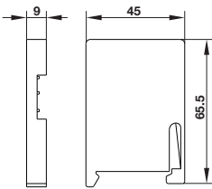
fig. 1. Abmessungen (mm)
