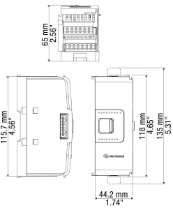
fig. 1. Dimensions (mm)
