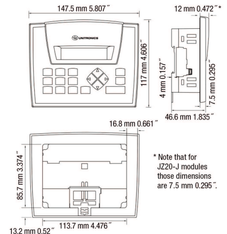
fig. 1. Dimensions (mm)
