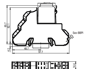
fig. 4. Abmessungen (mm)
