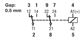
fig. 2. Wechselstrom-Schaltzyklen
