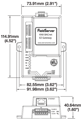
fig. 1. Dimensions (mm)
