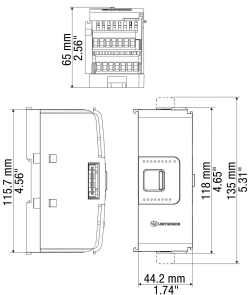
fig. 1. Dimensions (mm)
