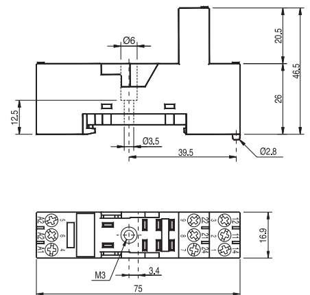
fig. 4. Dimensions (mm)
