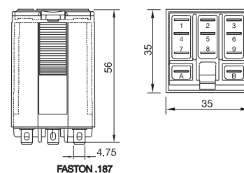
fig. 4. Abmessungen (mm)
