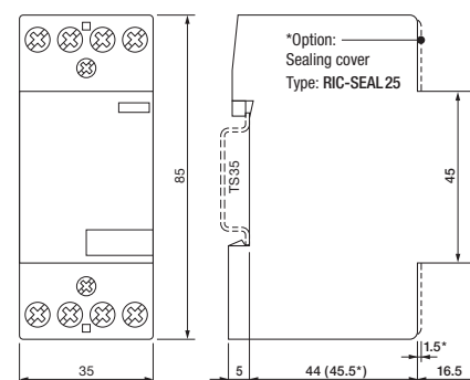
fig. 3. Abmessungen (mm)
