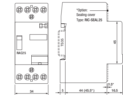
fig. 3. Dimensions (mm)
