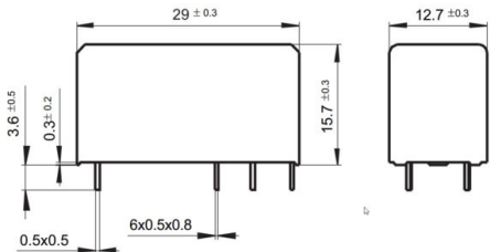
fig. 4. Dimensions (mm)
