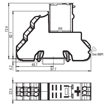
fig. 4. Abmessungen (mm)
