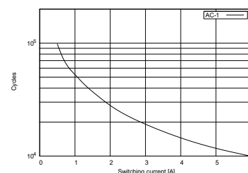
fig. 3. Gleichstrom-Grenzlastkurve
