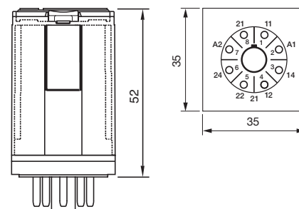
fig. 4. Dimensions (mm)
