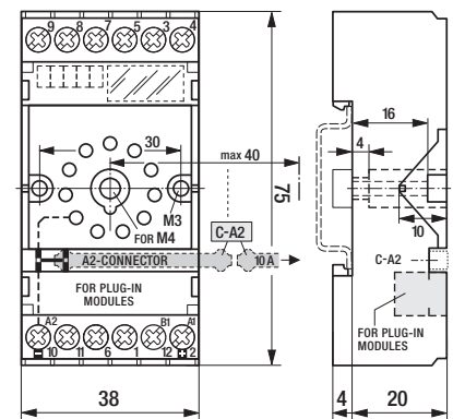
fig. 2. Abmessungen (mm)
