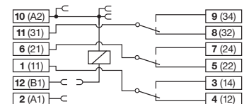
fig. 1. Verdrahtungsdiagramm
