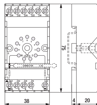
fig. 2. Abmessungen (mm)
