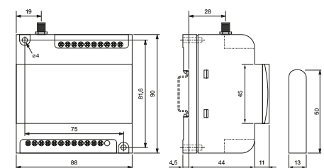
fig. 3. Dimensions (mm)
