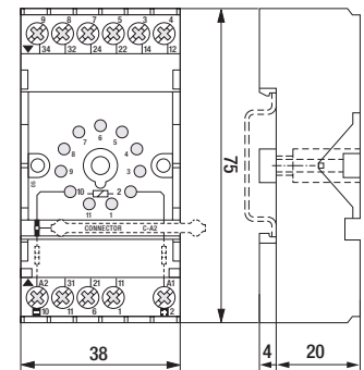
fig. 2. Abmessungen (mm)
