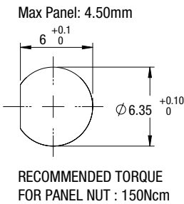
fig. 2. Abmessungen (mm)
