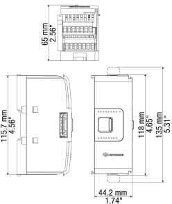
fig. 1. Dimensions (mm)
