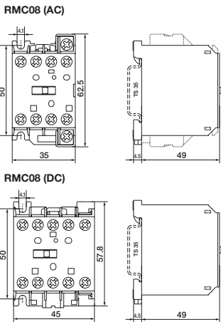
fig. 3. Dimensions (mm)
