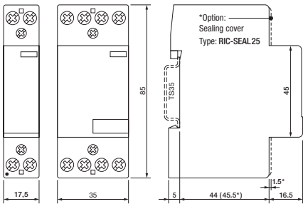
fig. 3. Dimensions (mm)
