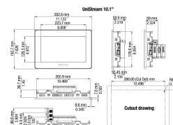
fig. 1. Dimensions (mm)
