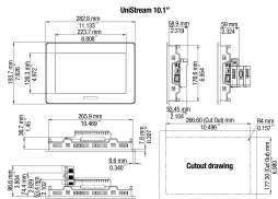
fig. 1. Dimensions (mm)
