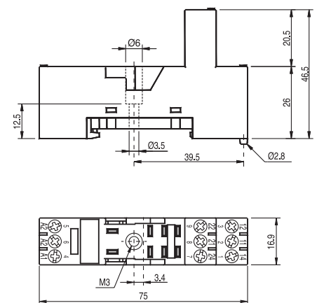
fig. 3. Dimensions (mm)
