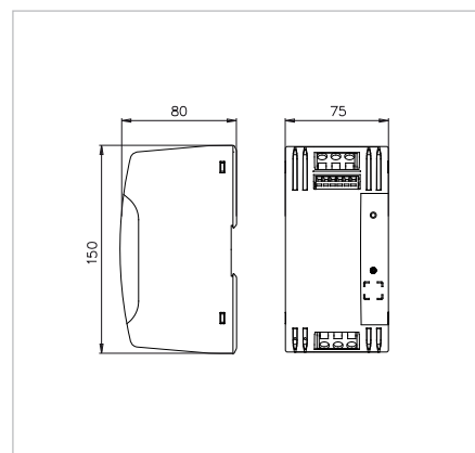
«Dimension drawing e» 75 mm module
