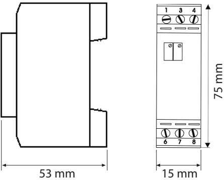
fig. 1. Dimensions (mm)
