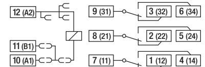
fig. 1. Verdrahtungsdiagramm
