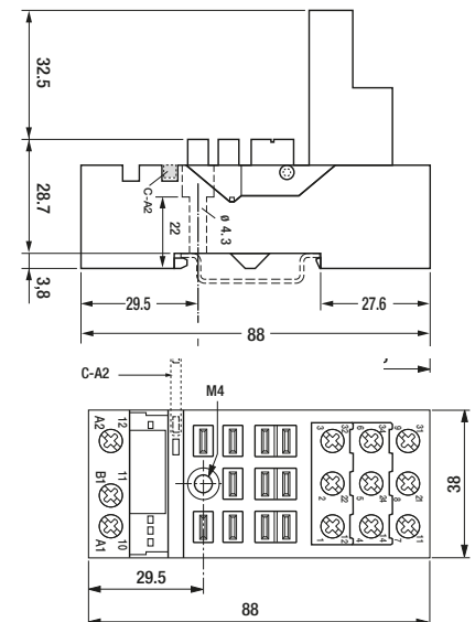
fig. 2. Abmessungen (mm)
