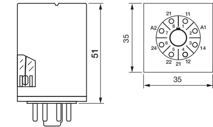
fig. 4. Dimensions (mm)
