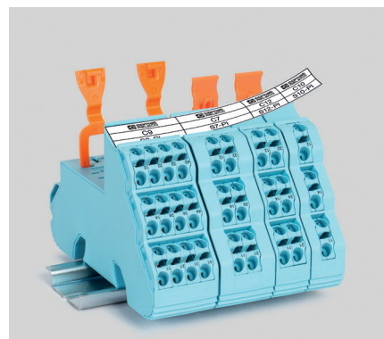
Mecanismo de encaje a presión para banda de marcado de 11 mm
