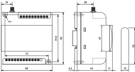
fig. 3. Dimensions (mm)
