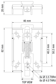
fig. 1. Dimensions (mm)
