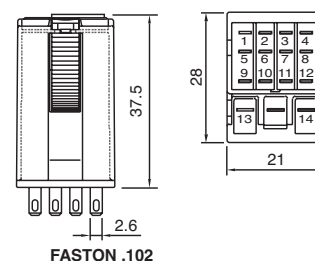
fig. 4. Dimensions (mm)
