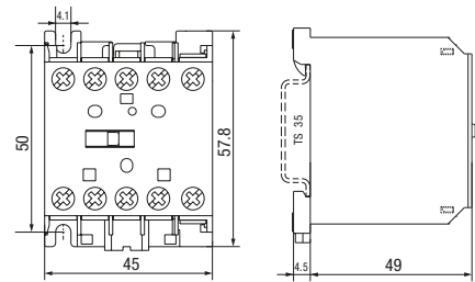
fig. 3. Dimensions (mm)
