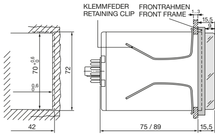
fig. 1. Dimensions (mm)
