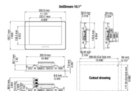
fig. 1. Dimensions (mm)
