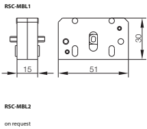
fig. 1. Dimensions (mm)
