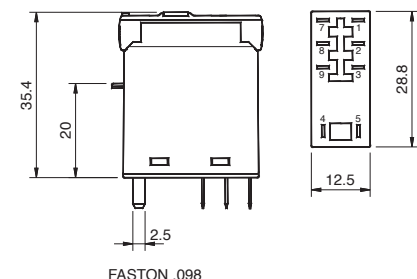
fig. 4. Dimensions (mm)
