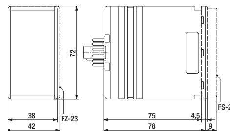
fig. 4. Abmessungen (mm)
