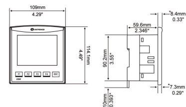
fig. 1. Abmessungen (mm)
