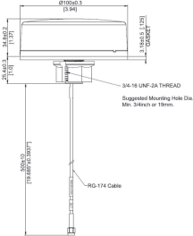
fig. 1. Dimensions (mm)
