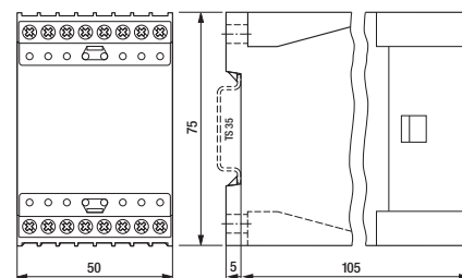
fig. 3. Dimensions (mm)
